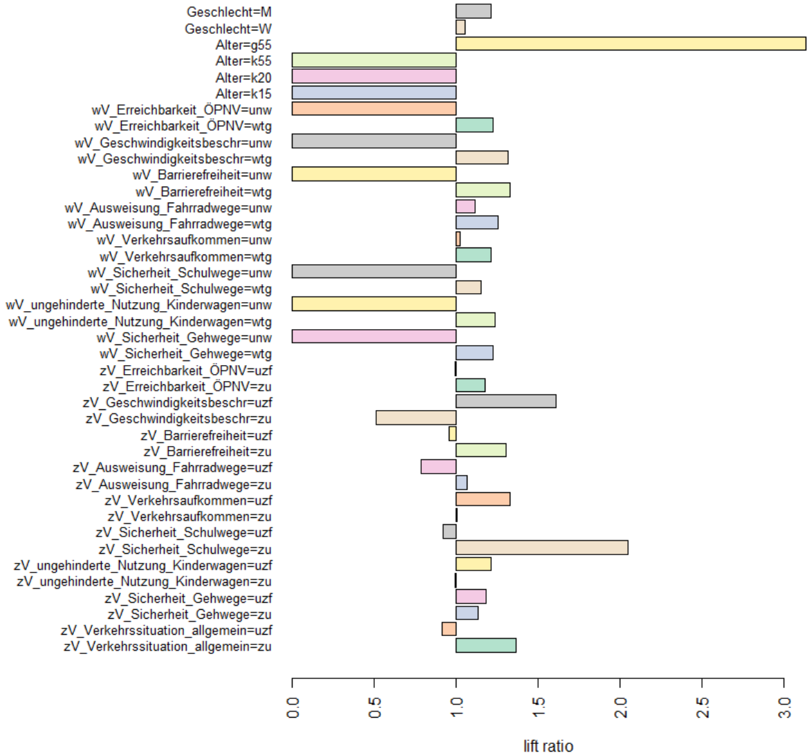
(Abbildung: FreqVG55.png)
